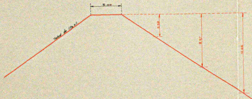
Perfil tipo en terraplen.
